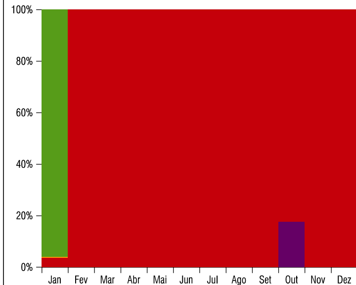
TEMPERATURA DO AR A 50m
