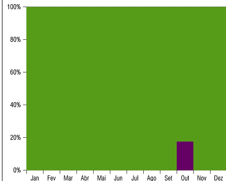
TEMPERATURA DO AR A 50m
